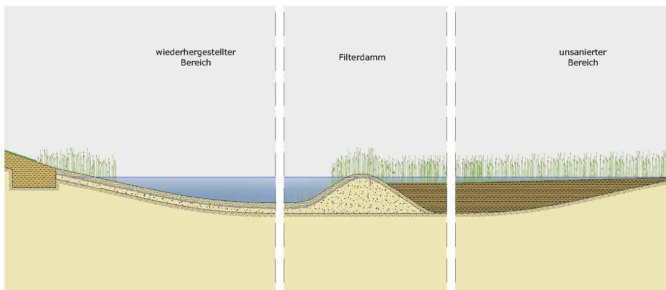
Schnitt durch den sanierten Pfuhl
