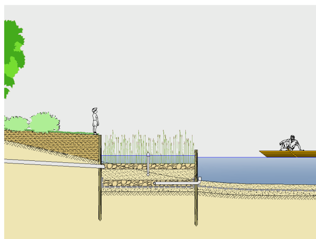
Bodenfilterschnitt
